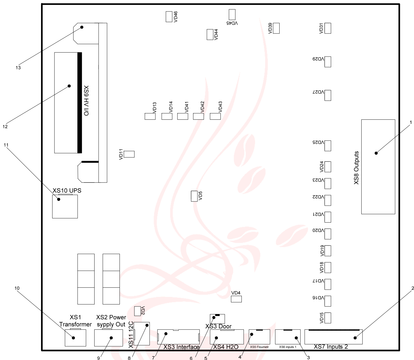
Рис. 7. Плата автоматики
